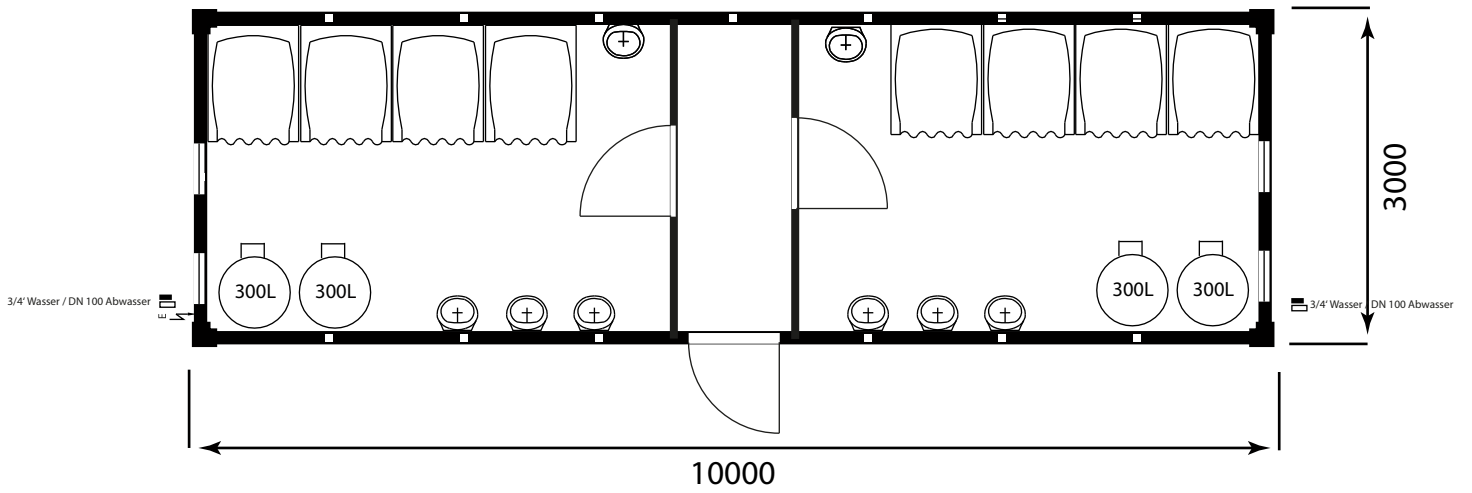
Containerrahmen 10000 x 3000
